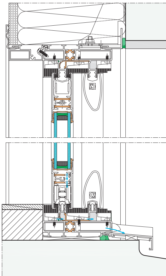
Coupe verticale
