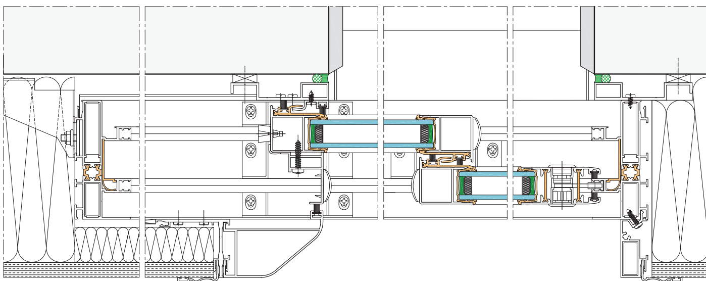
Coupe horizontale
